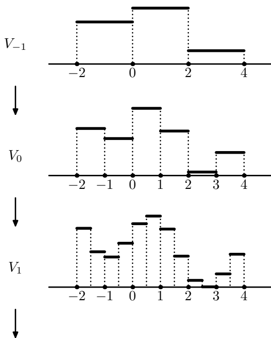
Рис. 3. КМА Хаара
