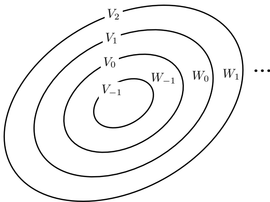
Рис. 5. Кратномасштабный анализ
