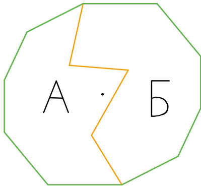
Рис. 6: Ломаная центрально-симметрична
